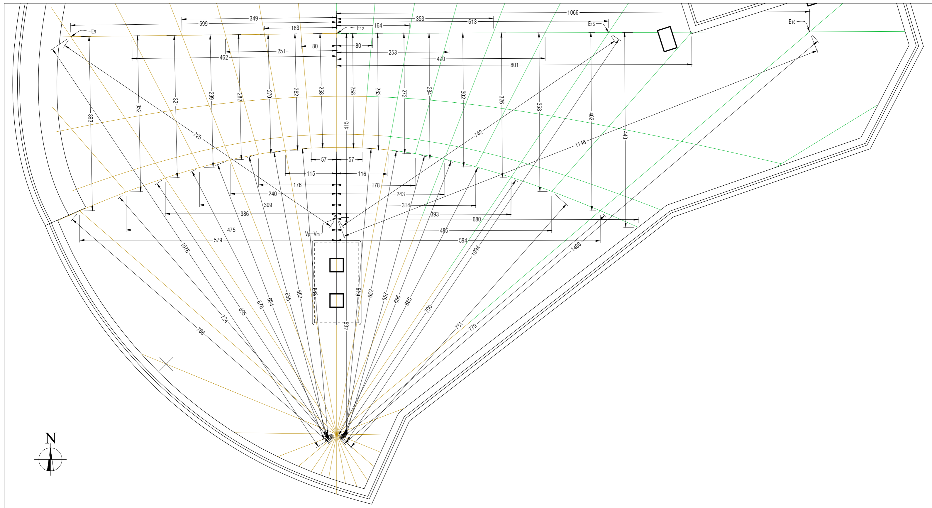
Individuazione del centro dell'orologio, dei punti d'ombra delle linee orarie e delle linee diurne solstiziale estiva ed equinoziale Planimetria (1:50)
