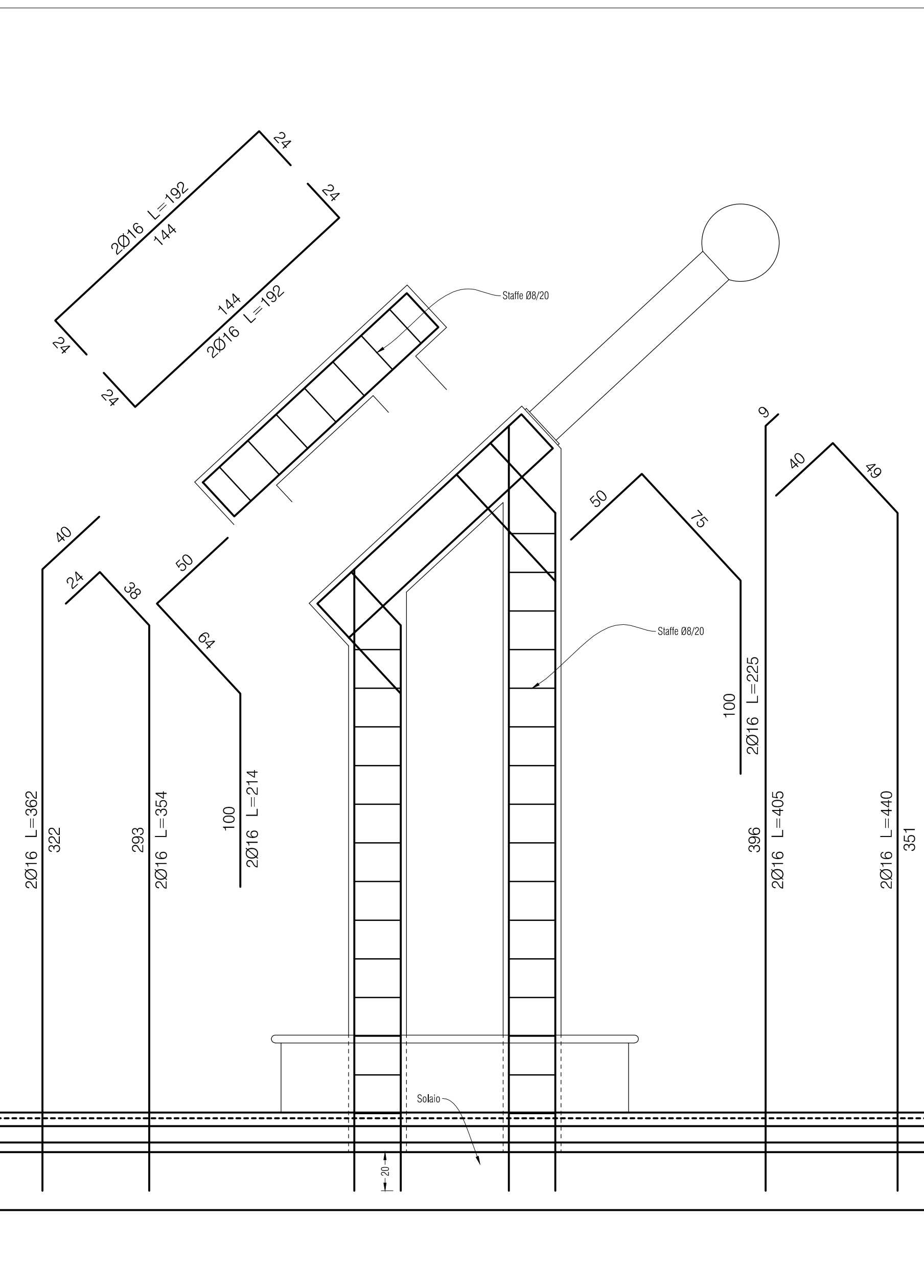
Prospetto est (1:20)
