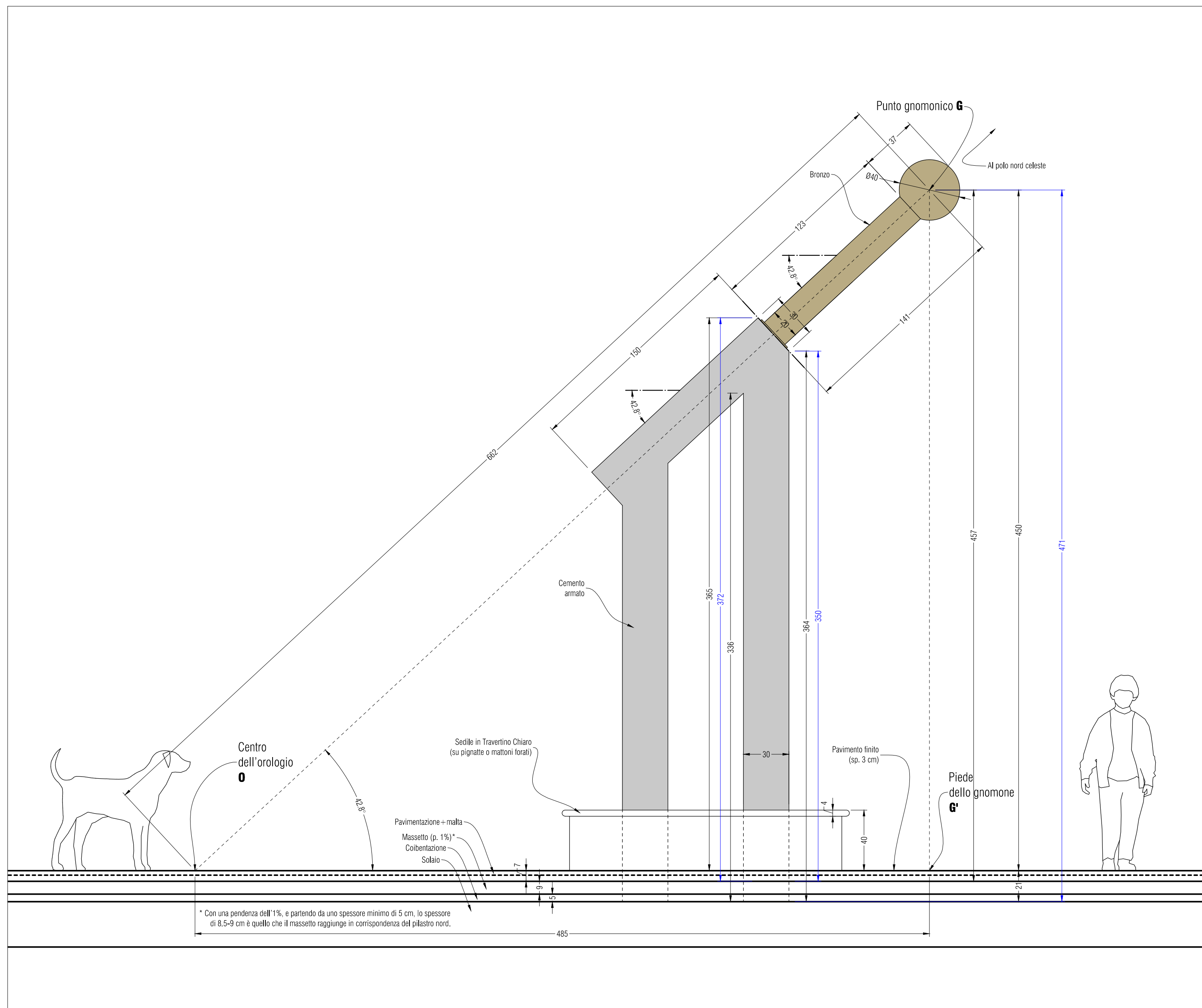
Prospetto est (1:20)
